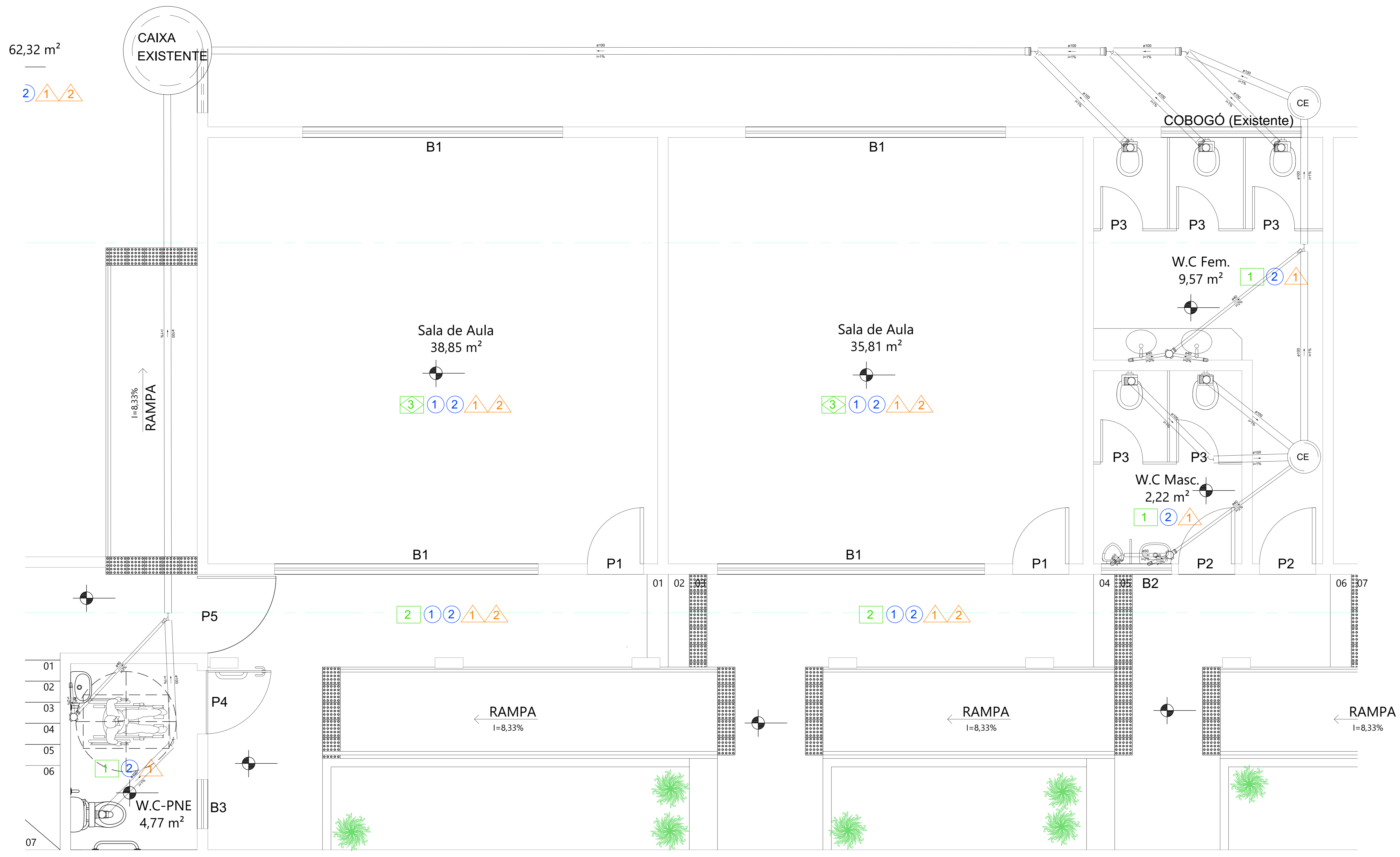
Detalhe S1 Escala 1:25
