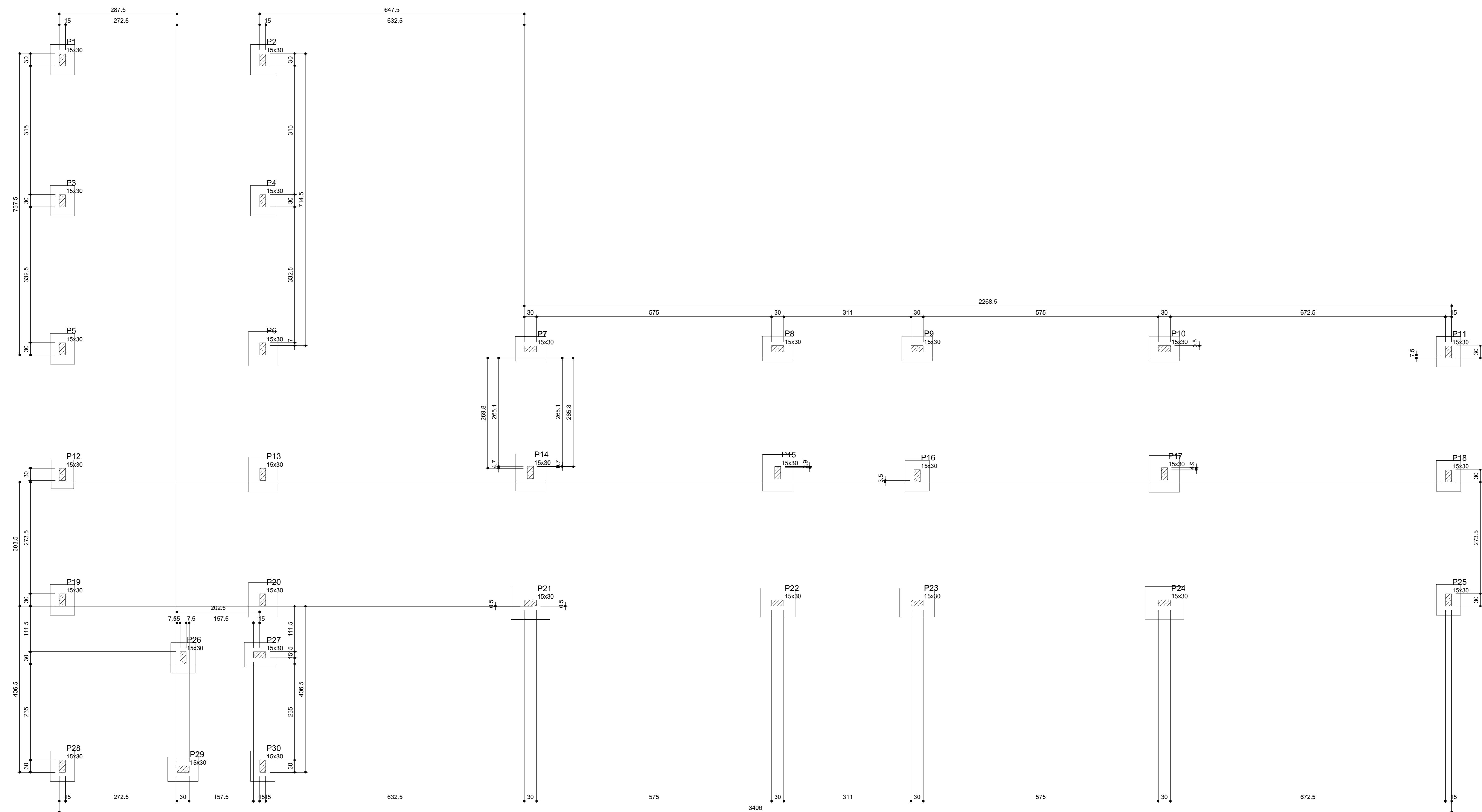
Forma do pavimento Fundação (Nível 0) escala 1:50
