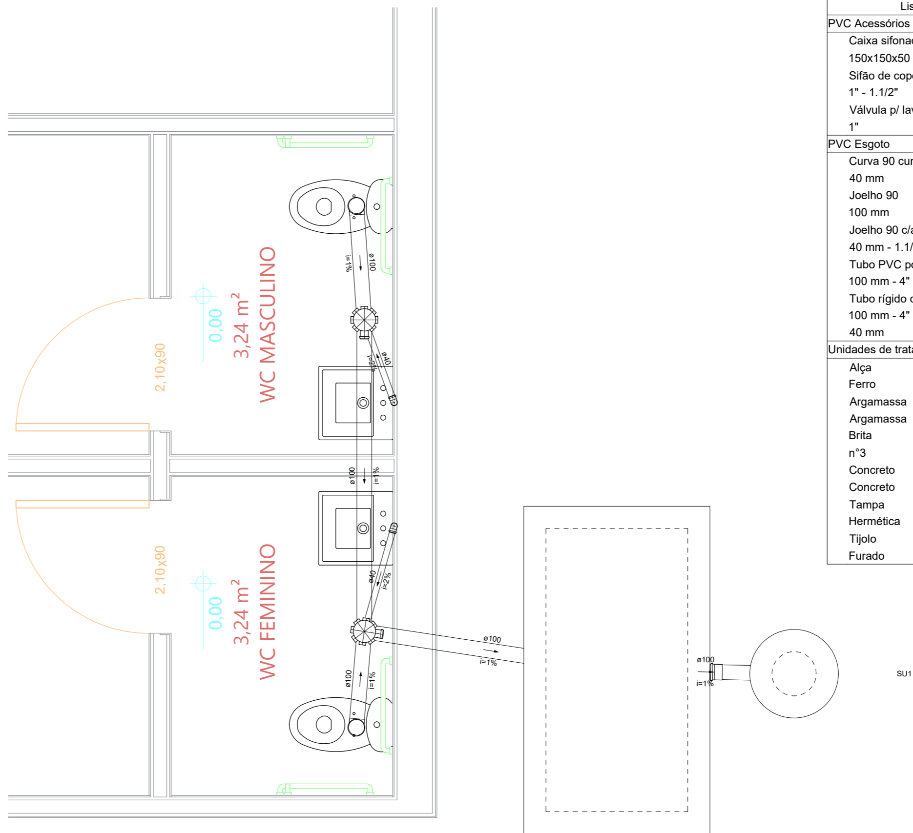
Detalhe S1 Escala 1:25
