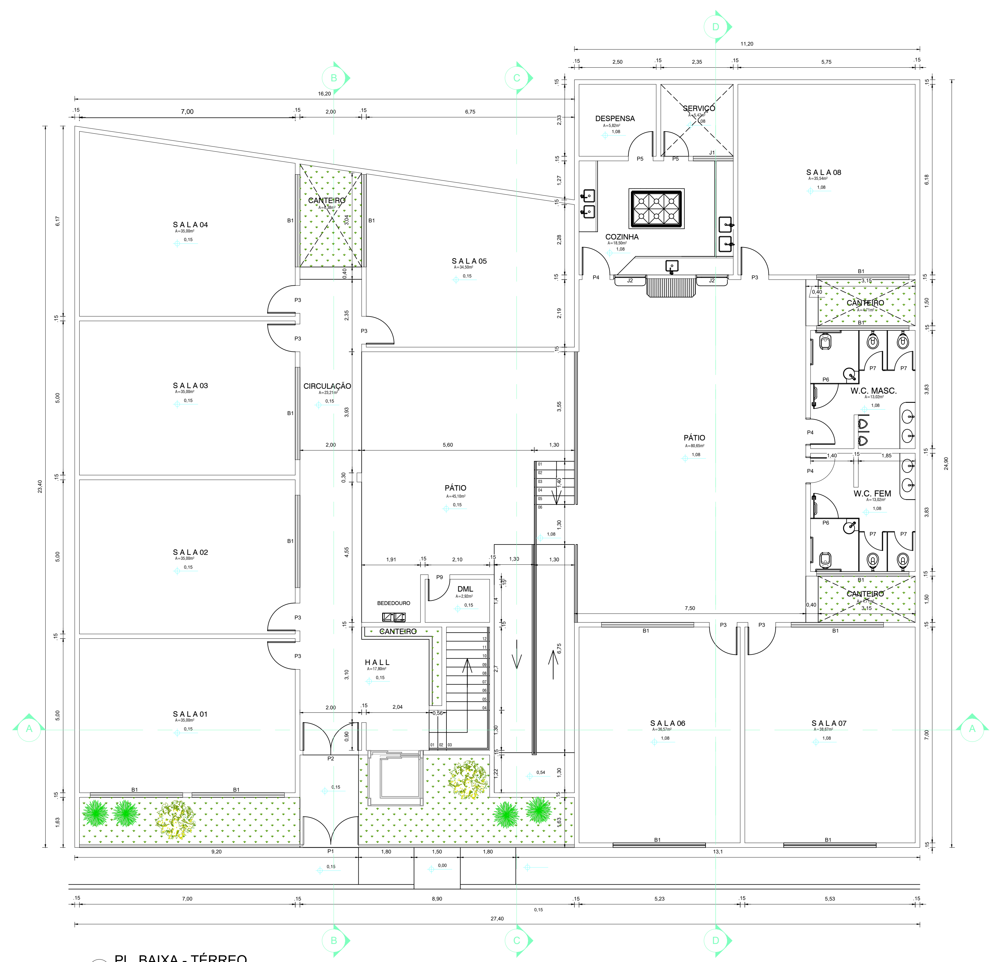
1 PL. BAIXA - TÉRREO 1:75
