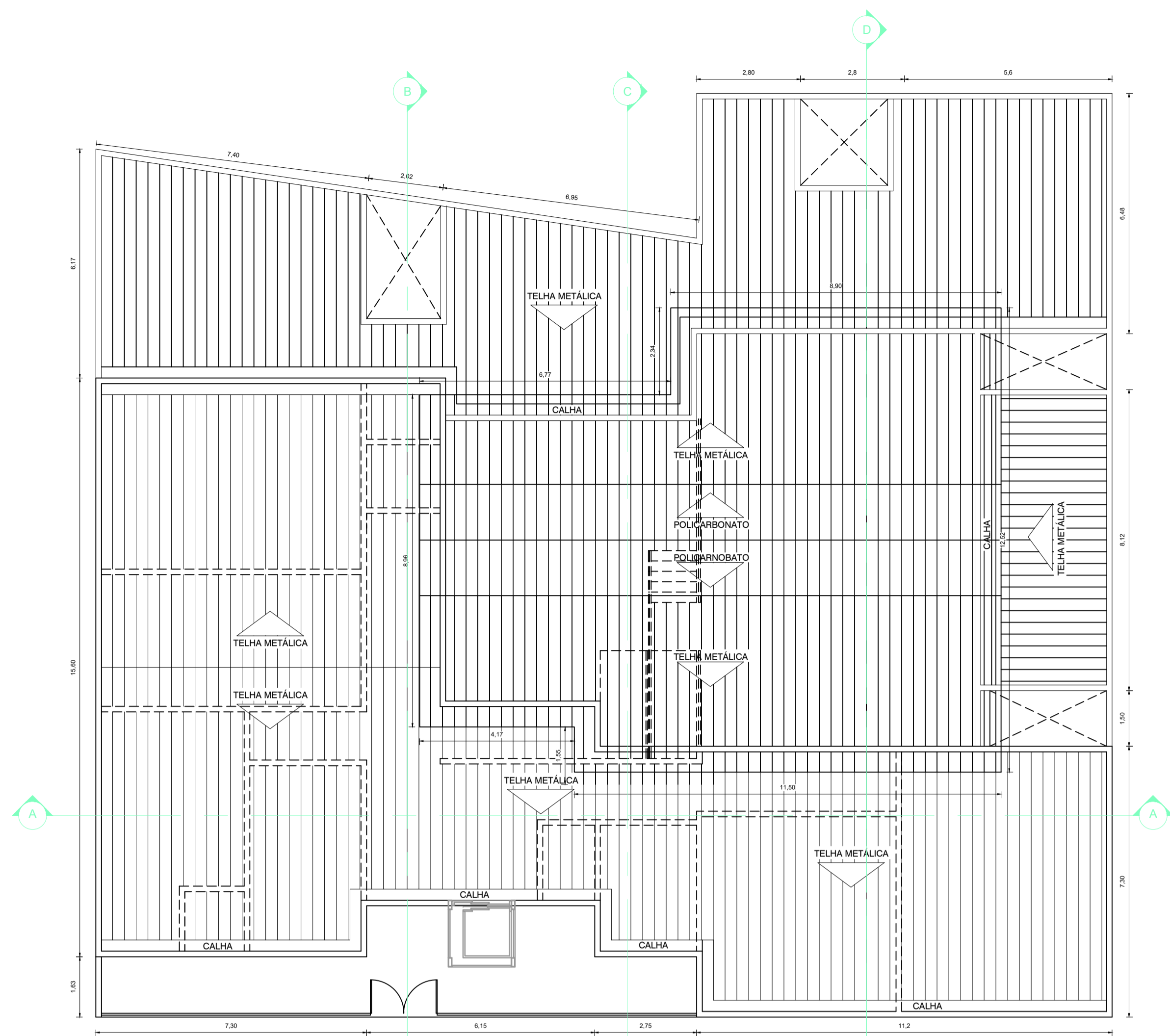
1 PL. BAIXA - COBERTURA 1 : 100
