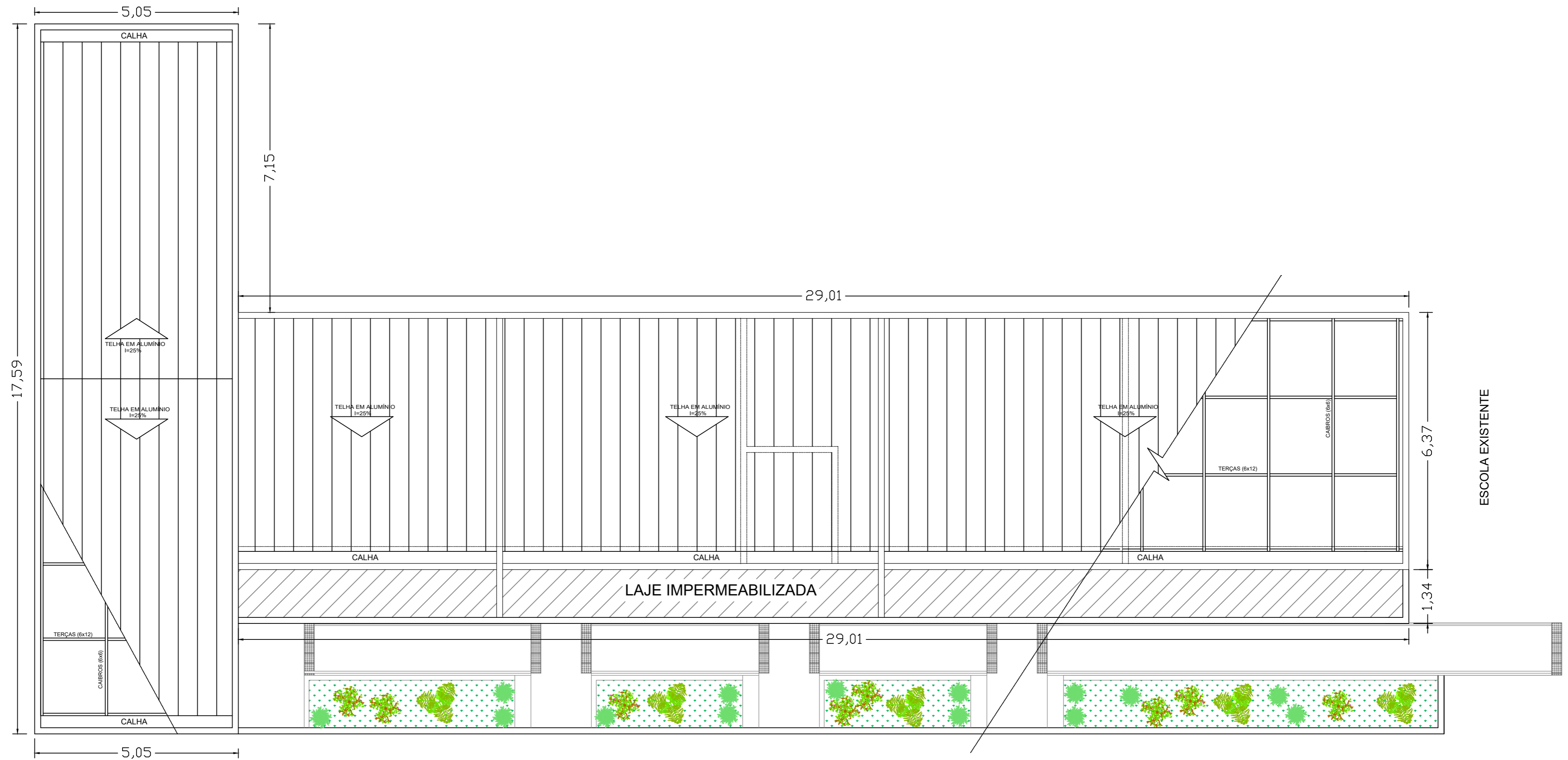
1 PL. BAIXA - COBERTURA 1 : 75
