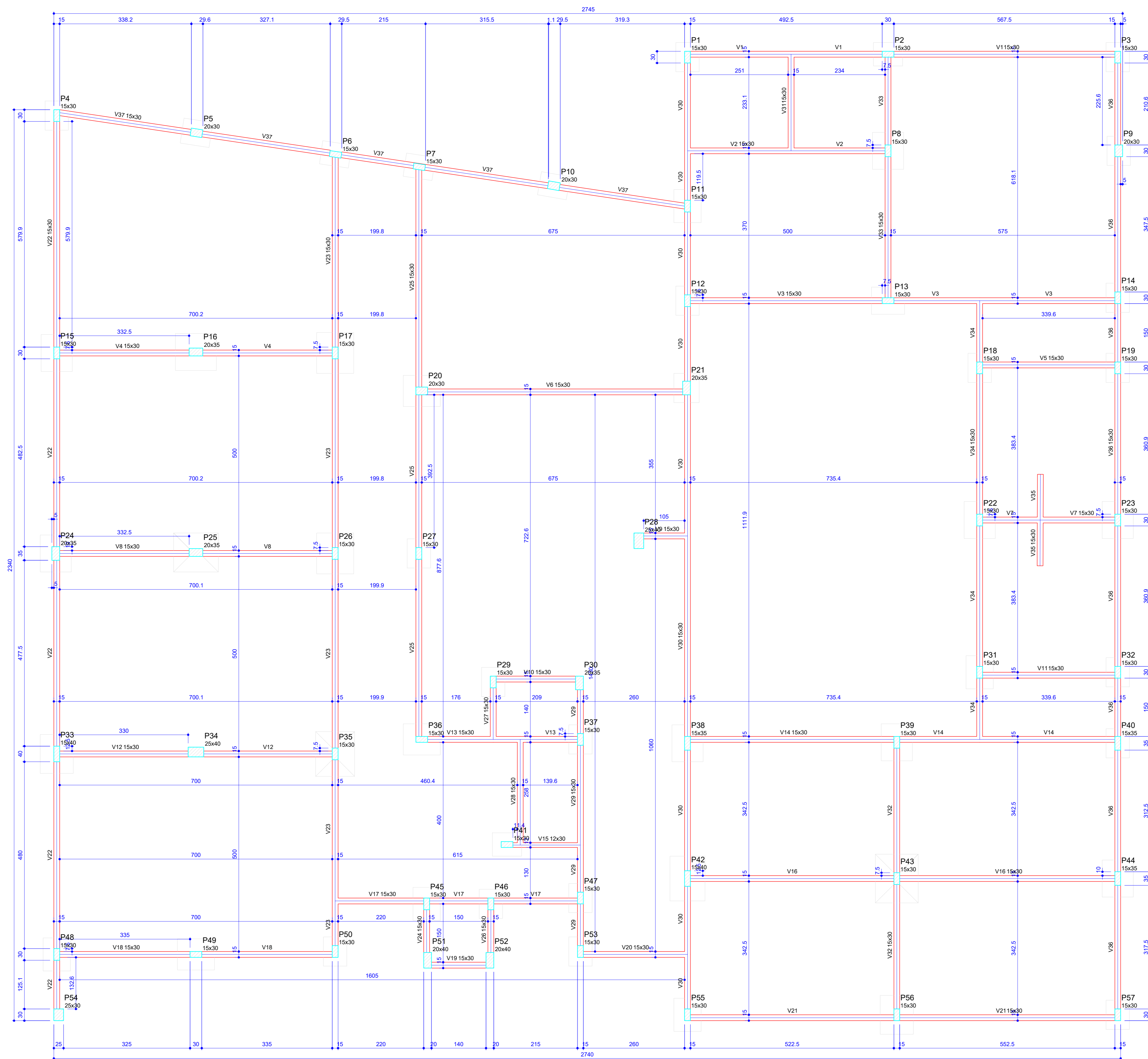
Forma do pavimento Fundação (Nível 0) escala 1:50
